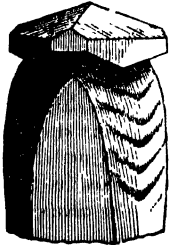
Calcite.
